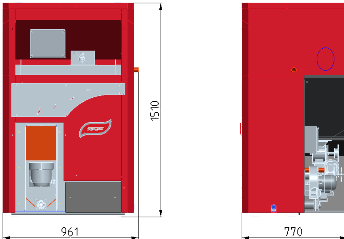
OPCIJA 3 Kotel Pellson X3 z oblogo brez polža in pokrovov – minimalna širina 770
