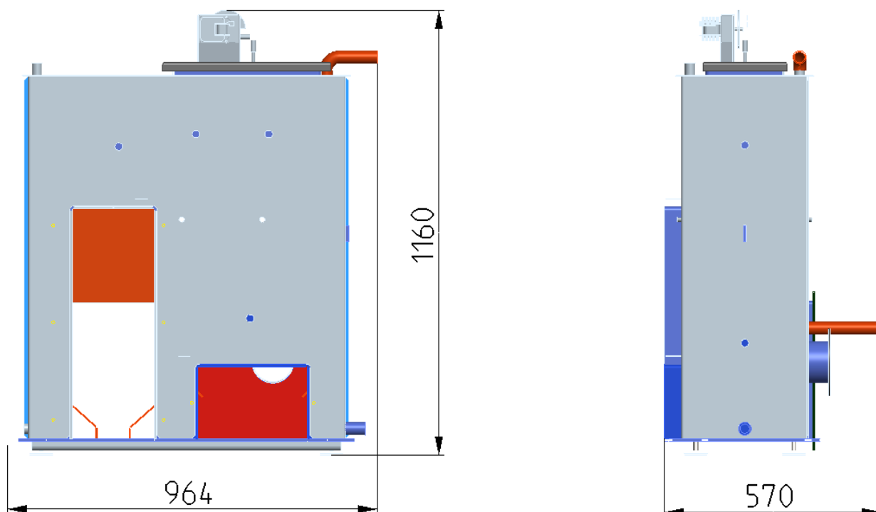
OPCIJA 4 Kotel Pellson X3 brez oblogo brez polža, pokrovov in gorilnika – minimalna širina 570
